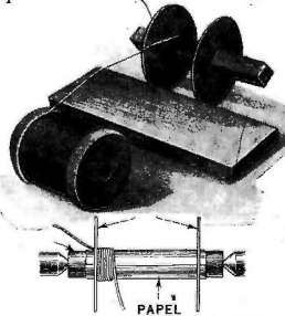
Fig. 4.—Cómo se inicia el enrollado del primario.—Sobre un tarugo de madera del mismo diámetro que el del interior del primario fundido, se enrollan dos o tres vueltas de papel corriente, bien barnizado con goma laca. Por ambos extremos se colocan dos discos de cartón, para que sirvan de soporte lateral al alambre y entonces se empieza el enrollado, dejando en el inicio unas 3 o 6 pulgadas para soldar a él la borna correspondiente.
