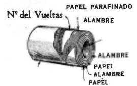
Fig. 5.—El primario terminado y listo para encajarlo en el secundario.
